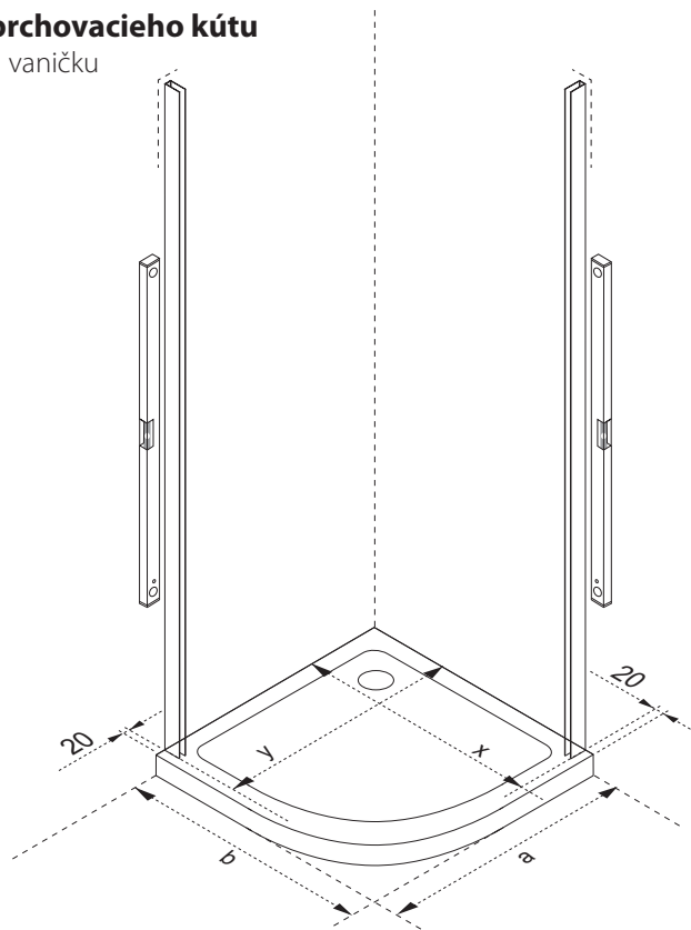
rozmery sprchovacieho kúta
