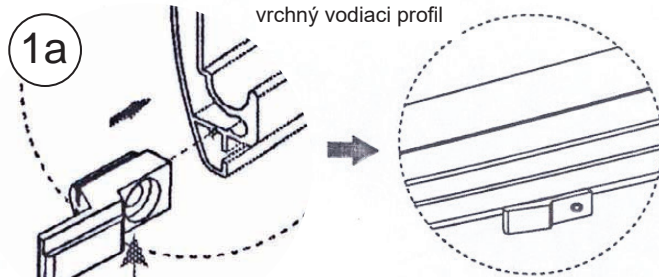
vrchný plastový úchyt pevného skla
