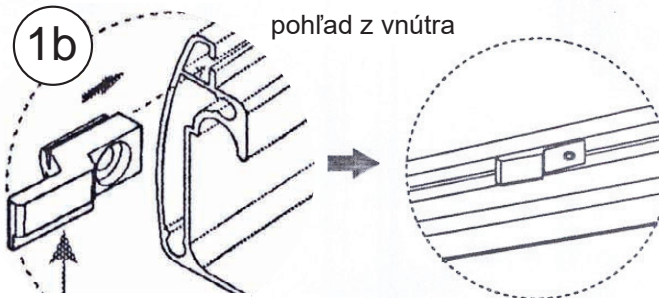
spodný vodiaci profil
