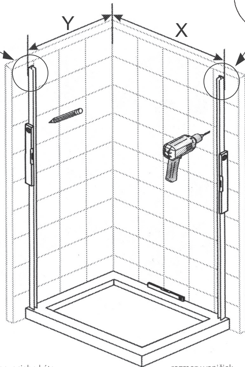
rozmery sprchovacieho kúta
